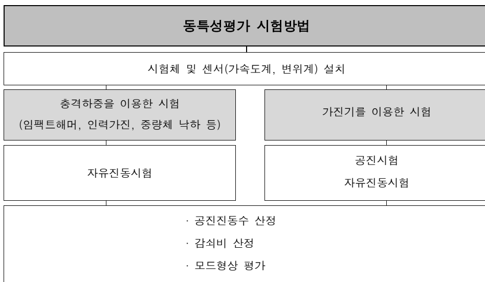
그림 1 - 동특성 평가 시험 방법 흐름도
